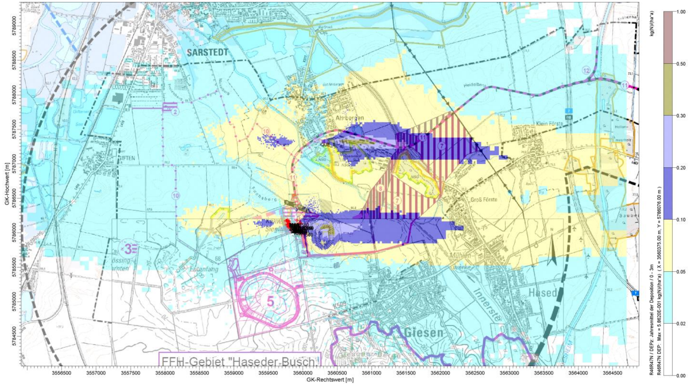
Variante 1: Jahresmittelwert der Immissionszusatzbelastung von Stickstoffdeposition durch das Hartsalzwerk Siegfried-Giesen in kg/(ha*a)
