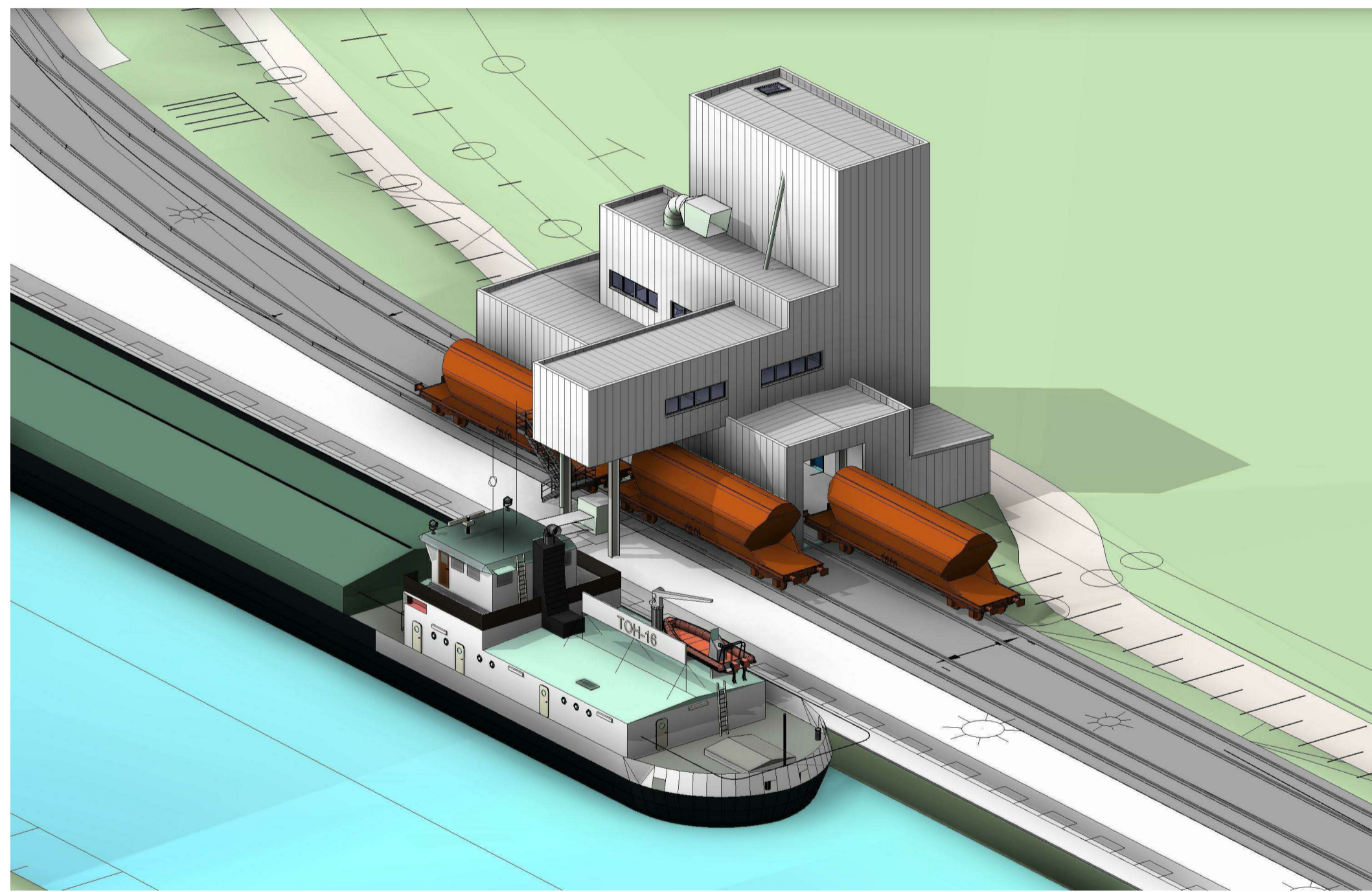
Isometrien Hafen Harsum
