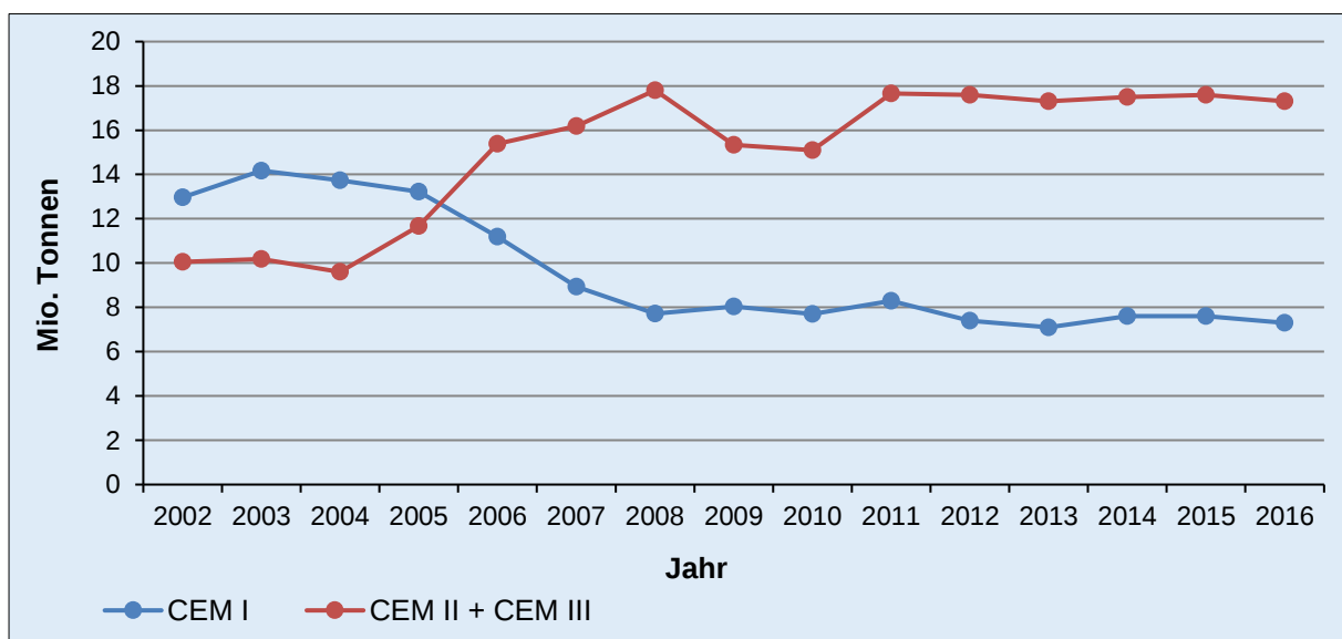
Abb. 5.4.2: Produktionsmengen von Zement nach CEM-Klassen in Deutschland 2002–2016 (Quelle: VDZ).
