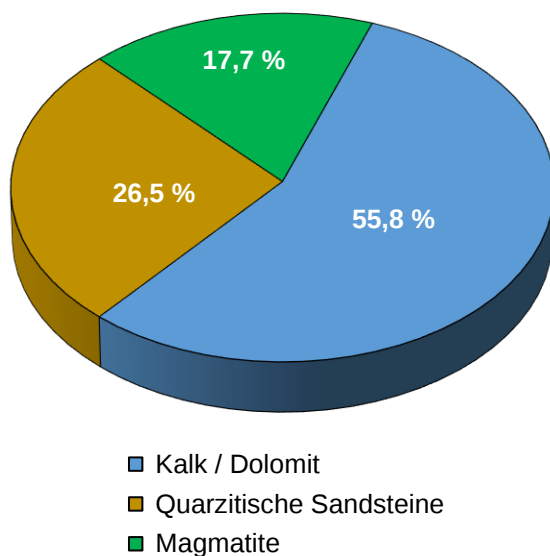
Abb. 5.3.3: Anteile verschiedener Gesteinsarten an der Natursteinproduktion Niedersachsens nach Angaben der Betriebe (Stand 2016).
