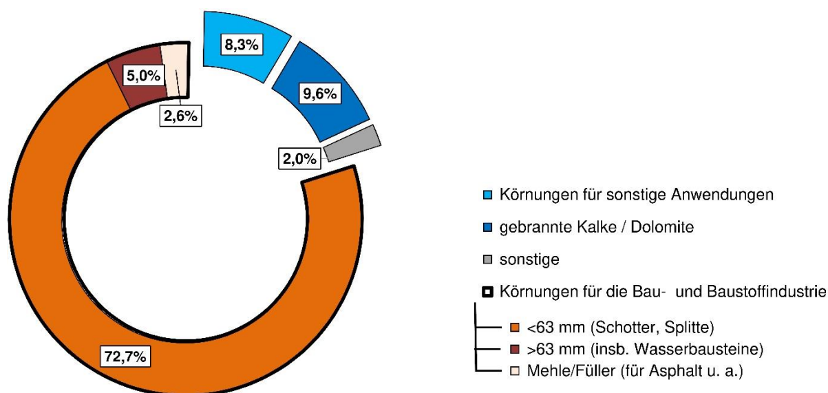
Abb. 5.3.6: Verwendungsbereiche von Natursteinen in Niedersachsen 2016 nach Betreiberangaben.
