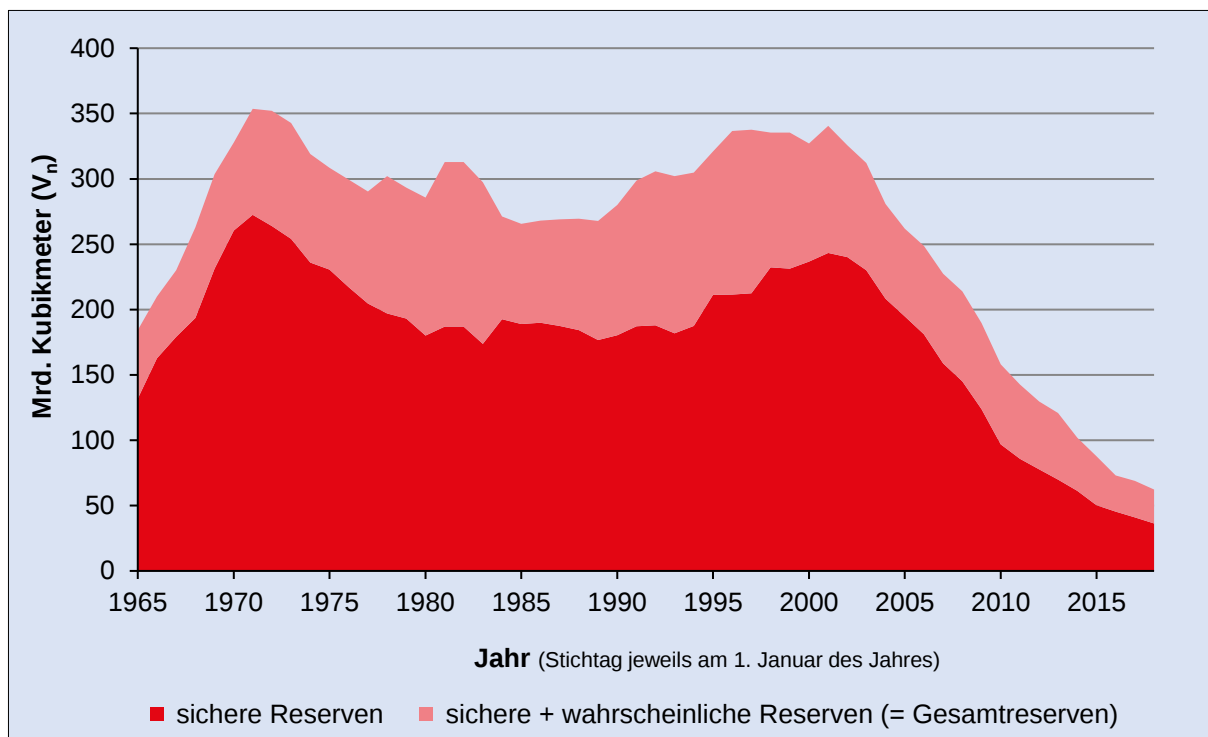
Abb. 3.1.5: Entwicklung der Erdgasreserven im Zeitraum von 1965 bis 2018 in Niedersachsen.
