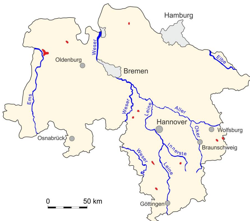
Abb. 5.1.14: Gebiete mit Quarzsanden (Industriesanden) in Niedersachsen.
