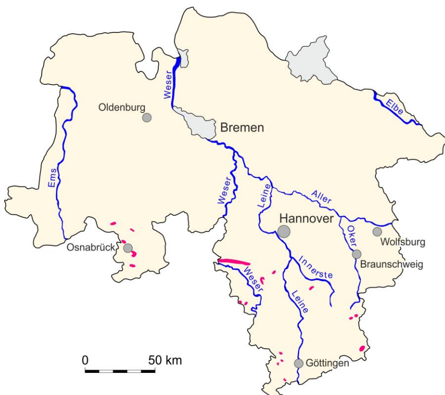
Abb. 5.3.1: Gebiete mit Naturstein-Vorkommen für Verkehrswege-, Beton- und Wasserbau in Niedersachsen.
