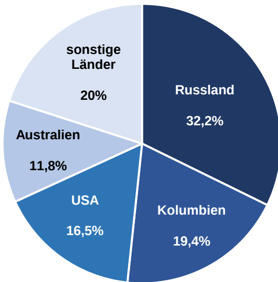
Abb. 7.8: Herkunft der Importkohle 2016 (Anteil der Lieferländer an den deutschen Steinkohleimporten).
