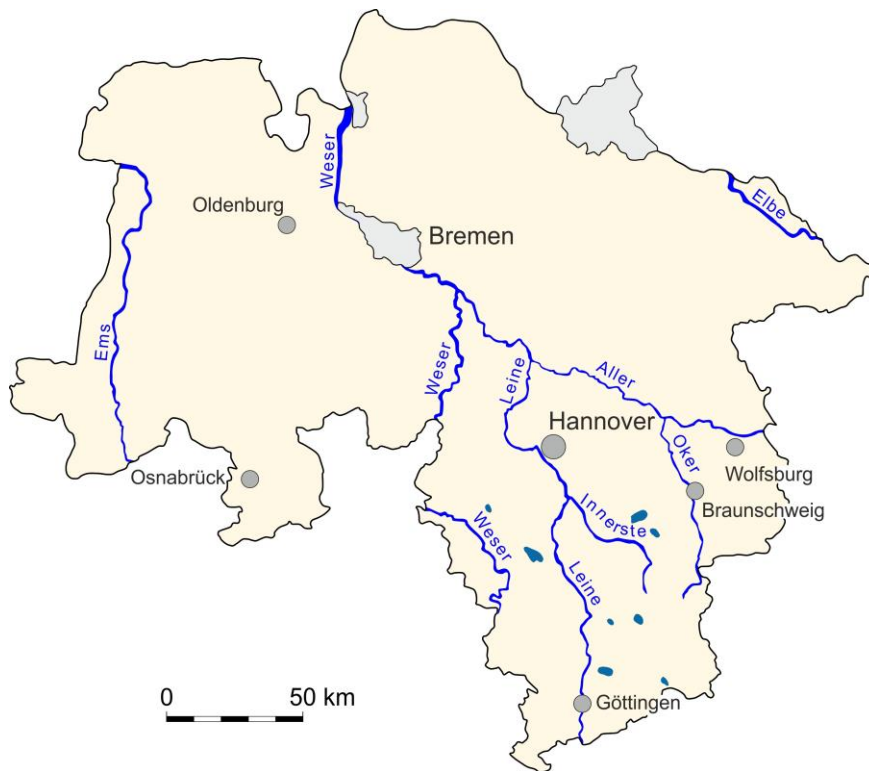
Abb. 5.3.2: Gebiete mit Vorkommen von Kalk- und Dolomitsteinen in Niedersachsen.
