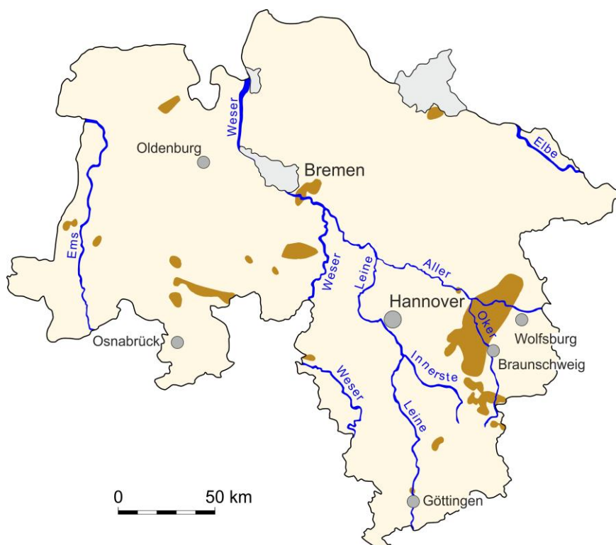
Abb. 3.3.1: Gebiete mit tief- liegenden Eisenerzlager- stätten in Niedersachsen.
