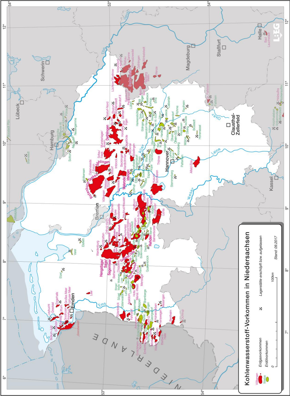
Abb. 3.1.1: Kohlenwasserstofflagerstätten in Niedersachsen.
