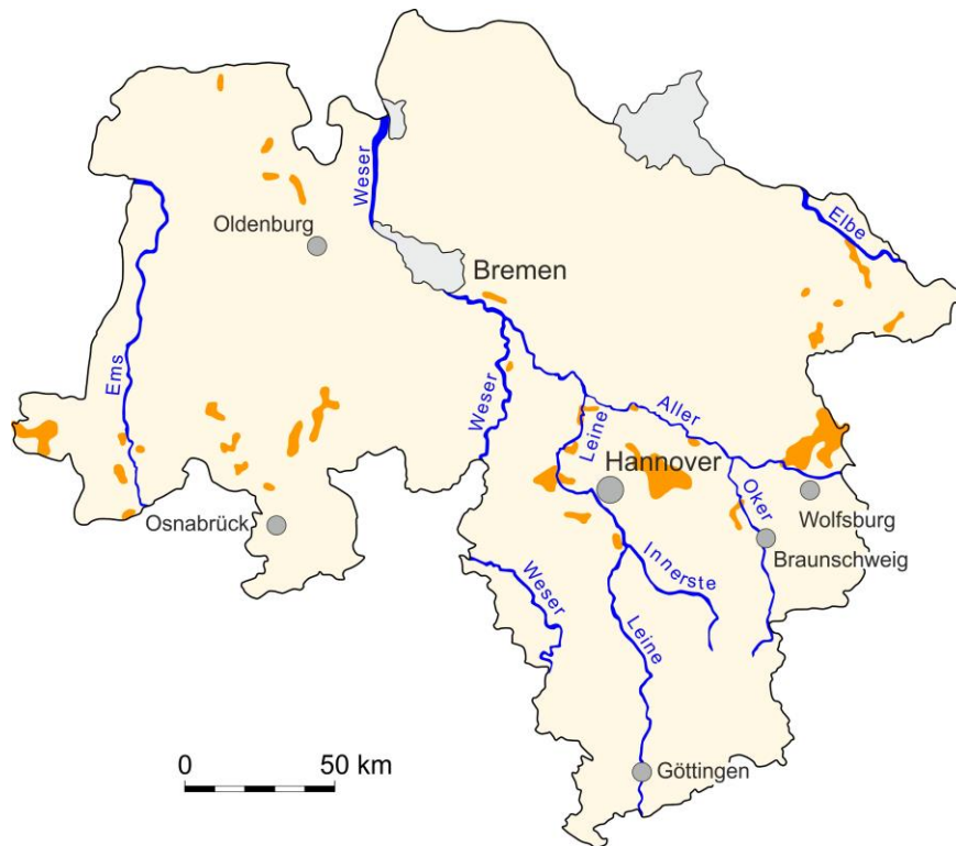
Abb. 5.1.2: Gebiete in Niedersachsen, in denen Grobsande dominieren oder häufiger auftreten.
