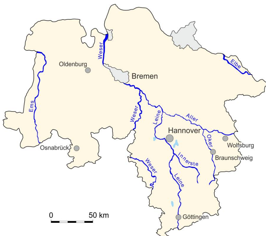
Abb. 5.4.1: Gebiete mit Vorkommen von Kalkmergelsteinen für die Zementindustrie in Niedersachsen.
