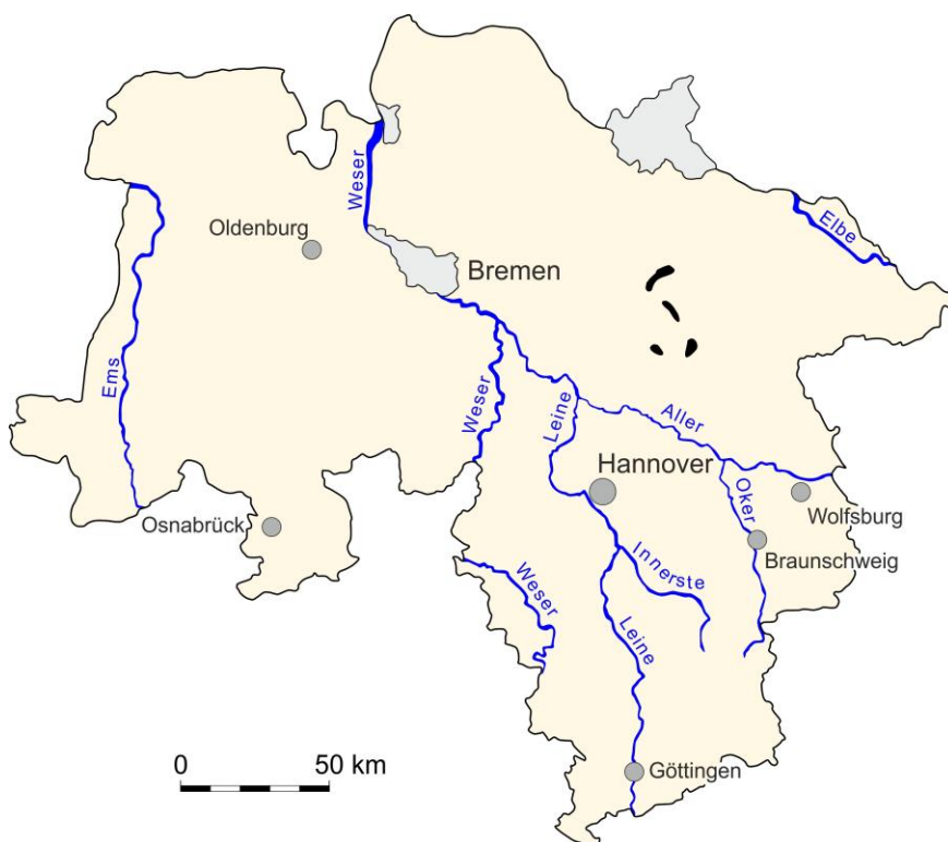
Abb. 5.7.1: Gebiete mit Kieselgur in Niedersachsen.
