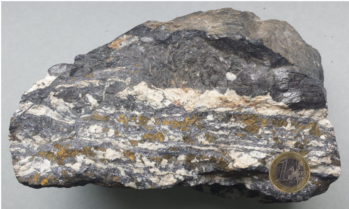
Abb. 3.3.2: Typisches Buntmetallerz der Lagerstätte bei Bad Grund im Harz, bestehend aus Bleiglanz (bleifarbig), Zinkblende (oben, bronzefarbig) und Kupferkies (goldfarbig) sowie Gangmittel aus Kalkspat (weiß). Sammlung LBEG/BGR Hannover.
