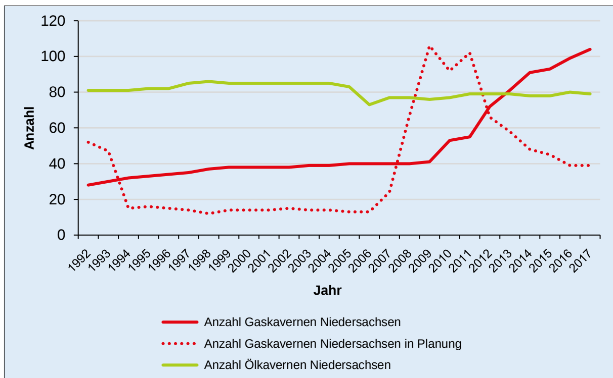
Abb. 3.2.5: Entwicklung der Anzahl von Salzkavernen zur Speicherung von Erdöl und Erdgas in Niedersachsen in der Zeit von 1992 bis 2017.
