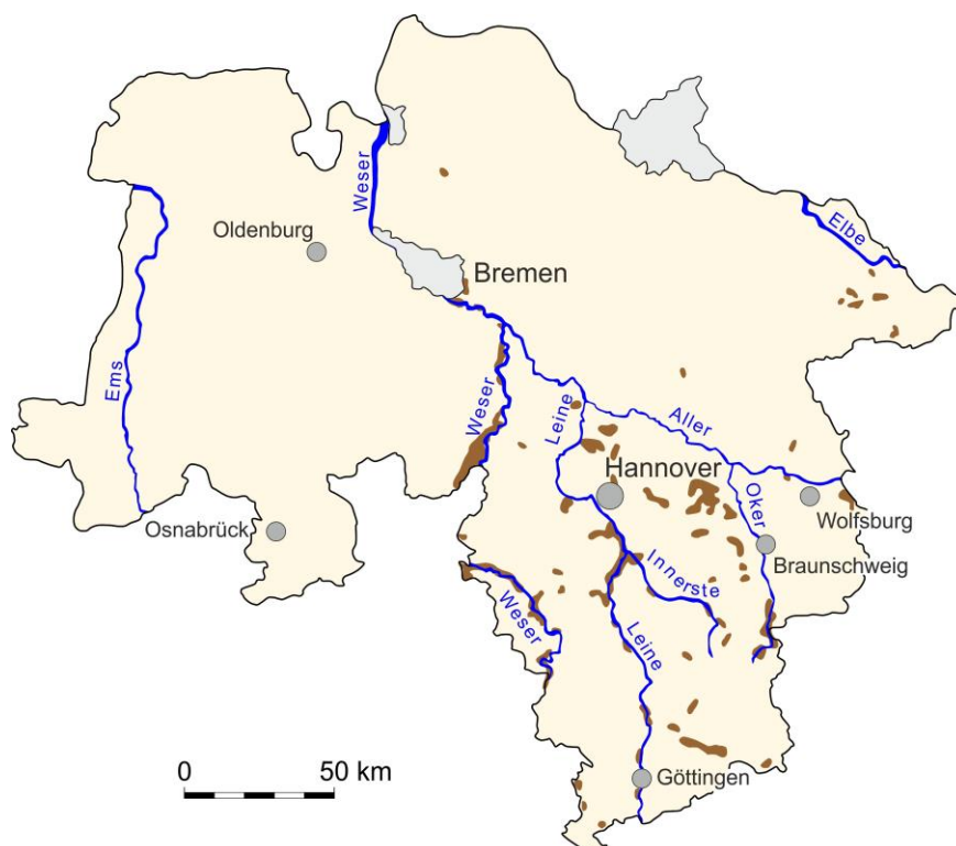
Abb. 5.1.1: Gebiete mit Kiesen und Kiessanden in Niedersachsen.
