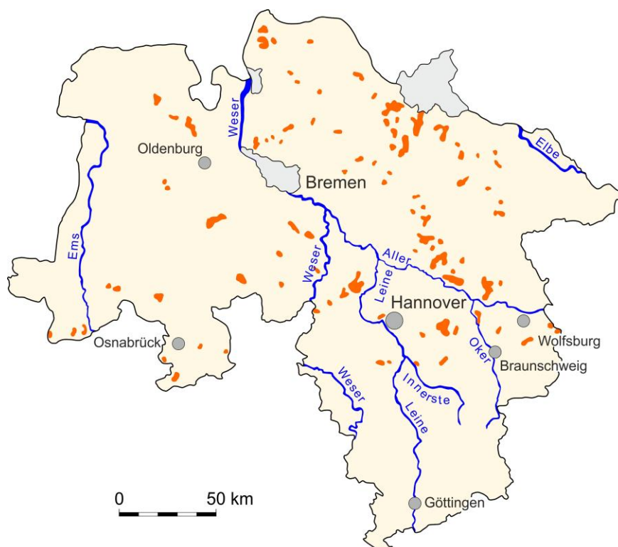
Abb. 5.1.3: Schwerpunkte der Verbreitung von Mittel- bis Feinsanden in Niedersachsen.
