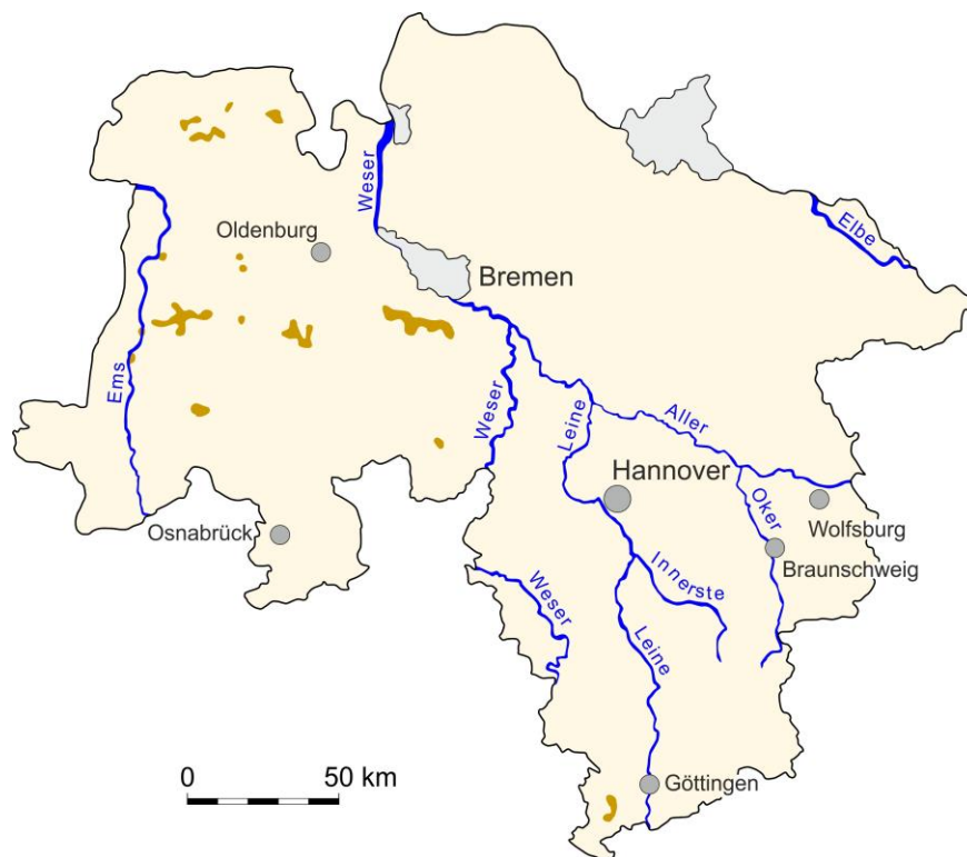
Abb. 5.1.4: Gebiete in Niedersachsen, in denen Feinsande dominieren.
