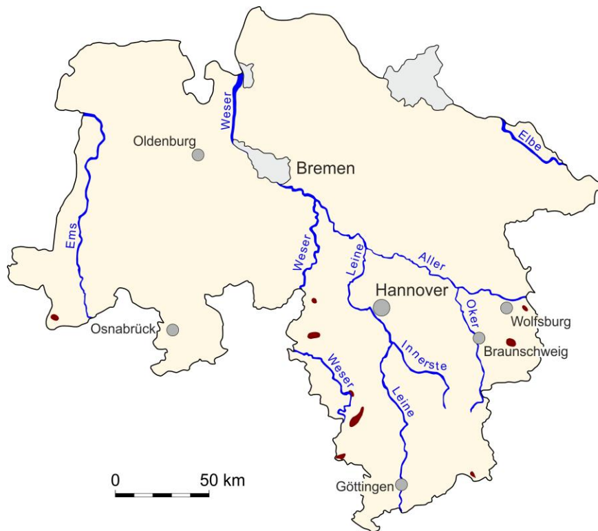
Abb. 5.6.2: Gebiete mit Vorkommen von Naturwerksteinen in Niedersachsen.
