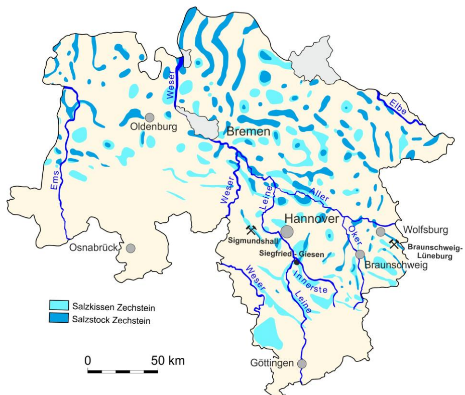
Abb. 3.2.1: Salzstöcke und -kissen in Niedersachsen.
