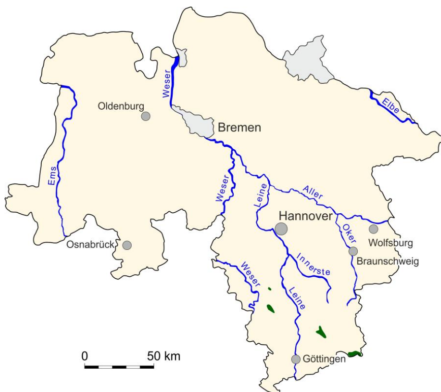
Abb. 5.5.1: Gebiete mit Vorkommen von Gips- und Anhydritsteinen in Niedersachsen.
