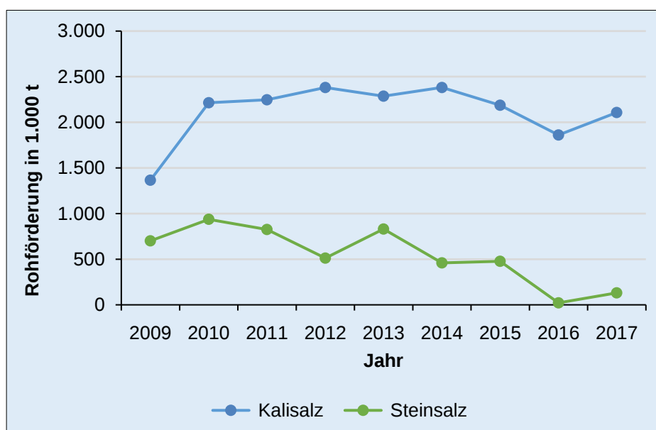
Abb. 3.2.2: Förderstatistik für Kali- und Steinsalz von 2009 bis 2017 für Niedersachsen.
