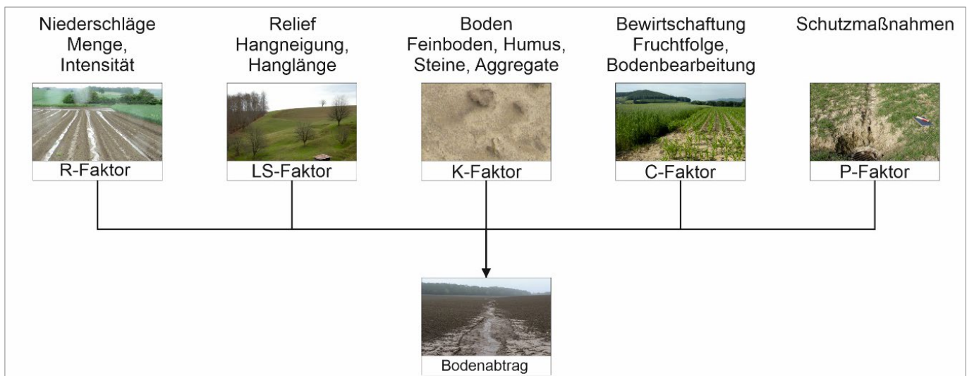
Abbildung 2: Faktoren der Allgemeinen Bodenabtragsgleichung (ABAG).
