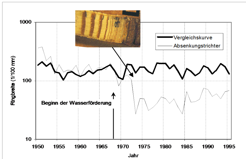
Abb. 3: Beispiel für abrupte Zuwachsreduktion von Unterstandsbäumen (= Absenkungstrichter) in einem Wasserentnahmehgebiet in Norddeutschland (aus WORBES & HILLMANN (2001), verändert). Die Bäume aus dem Unterstand reagieren auf den Beginn der Wasserförderung, die in der Nähe der Brunnenreihe von deutlichen Absenkungen des Grundwassers um mehrere Meter begleitet ist. Zum Vergleich der Verlauf einer Vergleichskurve, die von nicht beeinflussten Bäumen gebildet wurde.
