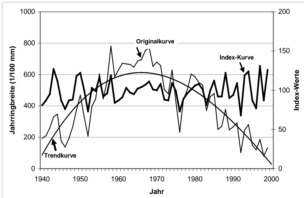
Abb. 1: Darstellung von Originaldaten, einer dazugehörigen Trendkurve (hier eine polynomische Ausgleichskurve 2. Ordnung) und der indextierten Kurve, deren Werte um den Mittelwert 100 normalverteilt sind. Die Trendkurve zeigt die langfristige Wachstumsentwicklung, wie z. B. zunehmende Lichtkonkurrenz, die Indexkurve zeigt die Schwankungen von Jahr zu Jahr, die in erster Linie klimainduziert sind. Man beachte, dass die jährlichen Schwankungen in Original- und Trendkurve identisch verlaufen (WORBES 2004).
