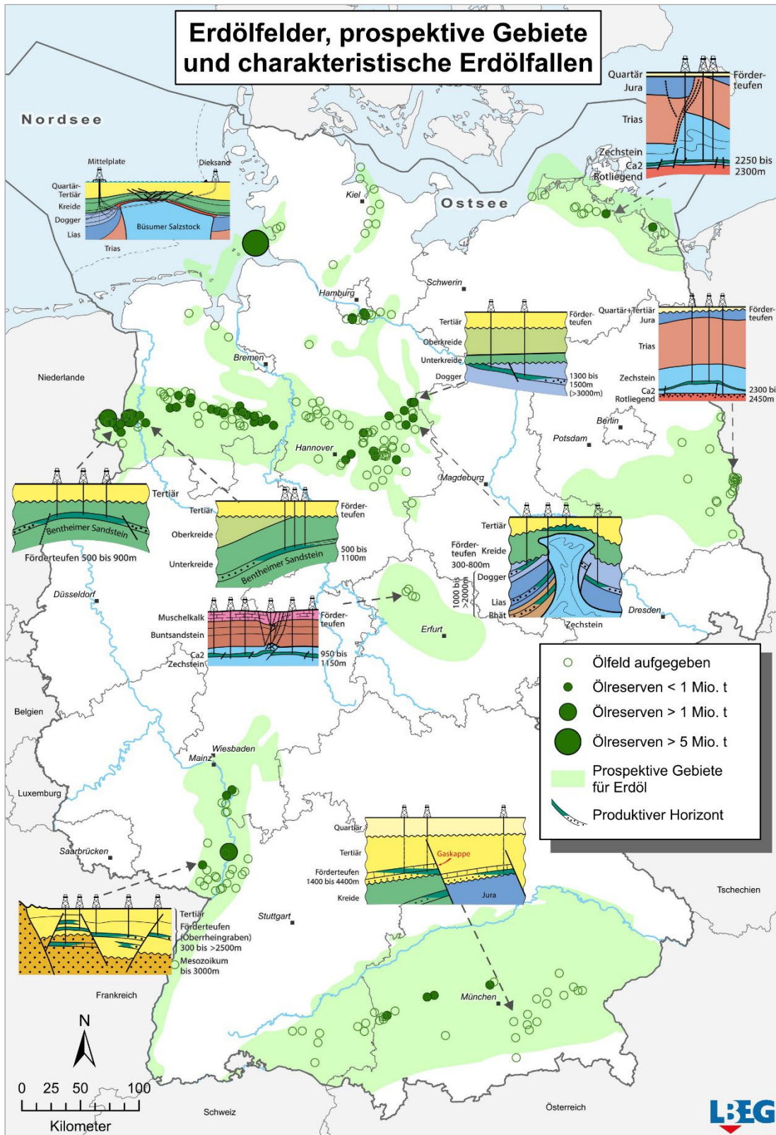
Anl. 3: Erdölfelder, prospektive Gebiete und charakteristische Erdölfallen am 01.01.2023.
