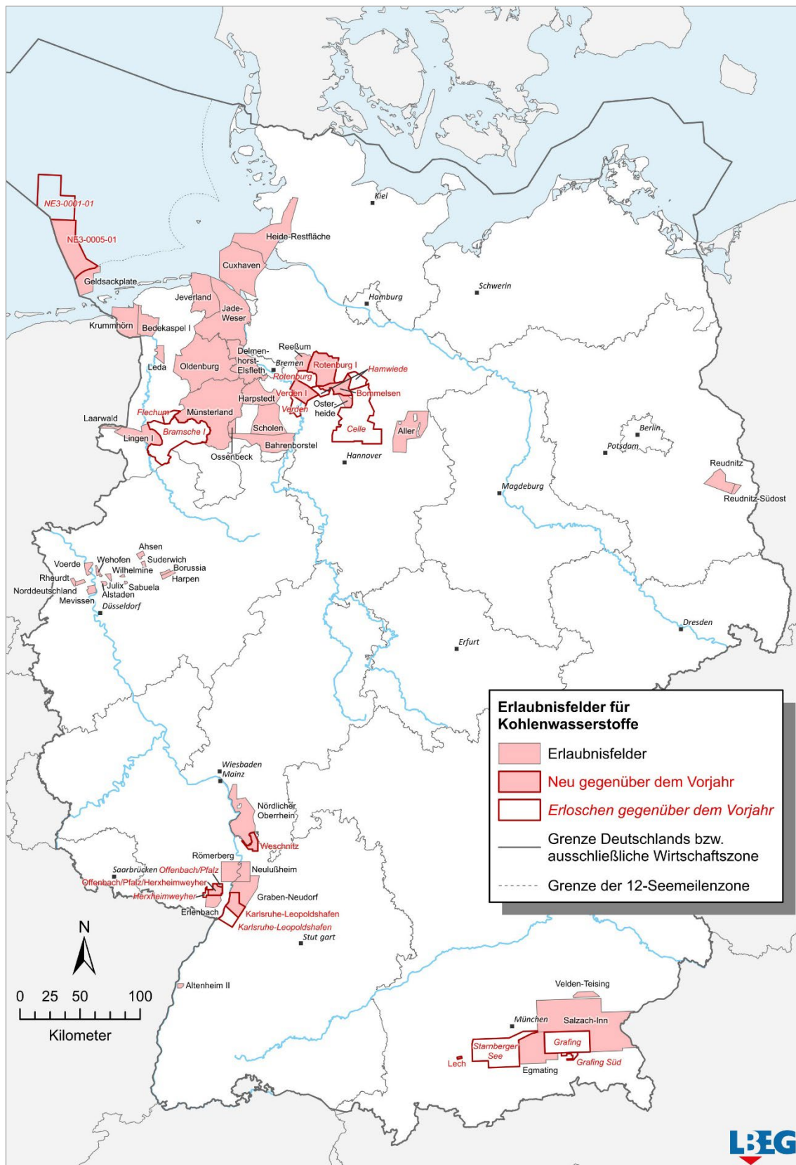
Abb. 4: Erlaubnisfelder für Kohlenwasserstoffe, Stand 31.12.2022 (Quelle: zuständige Bergverwaltungen).
