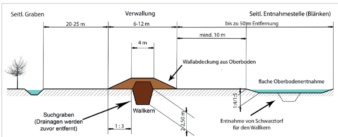
Abb. 4.9: Skizze zum Bau einer Torfdichtwand. Damm nach dem System Ehlers/Mordhorst-Bretschneider (MORDHORST-BRETSCHNEIDER 2018).
