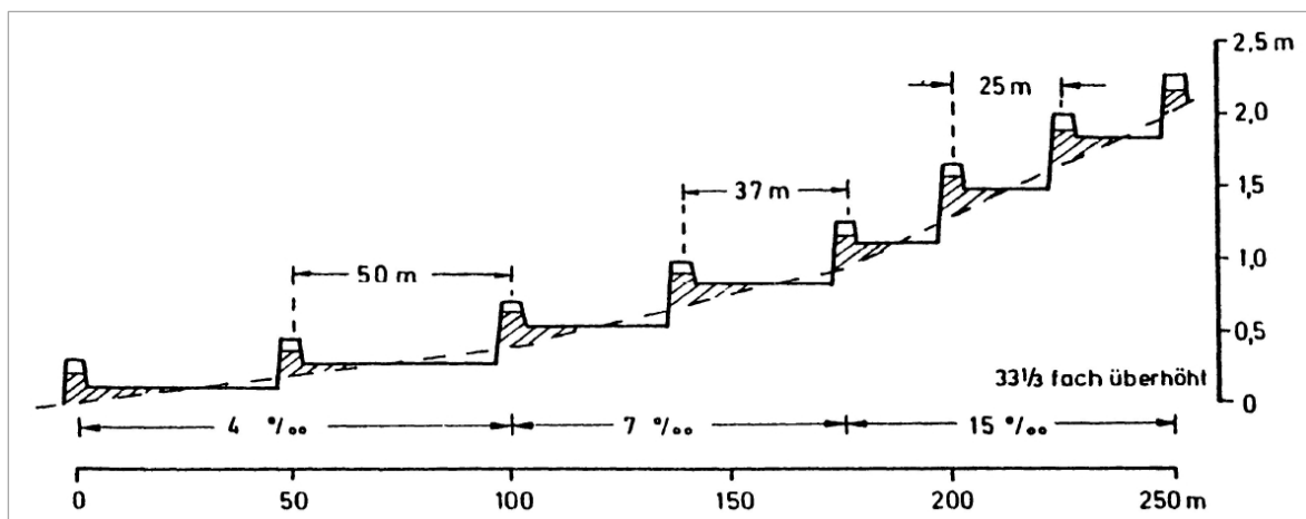
Abb. 4.5: Ökotechnisches Schema zur Hochmoorregeneration bei geneigter Moorfläche (= Niederschlagsretention mittels Überstau-Verfahren; EGGELSMANN (1987)).
