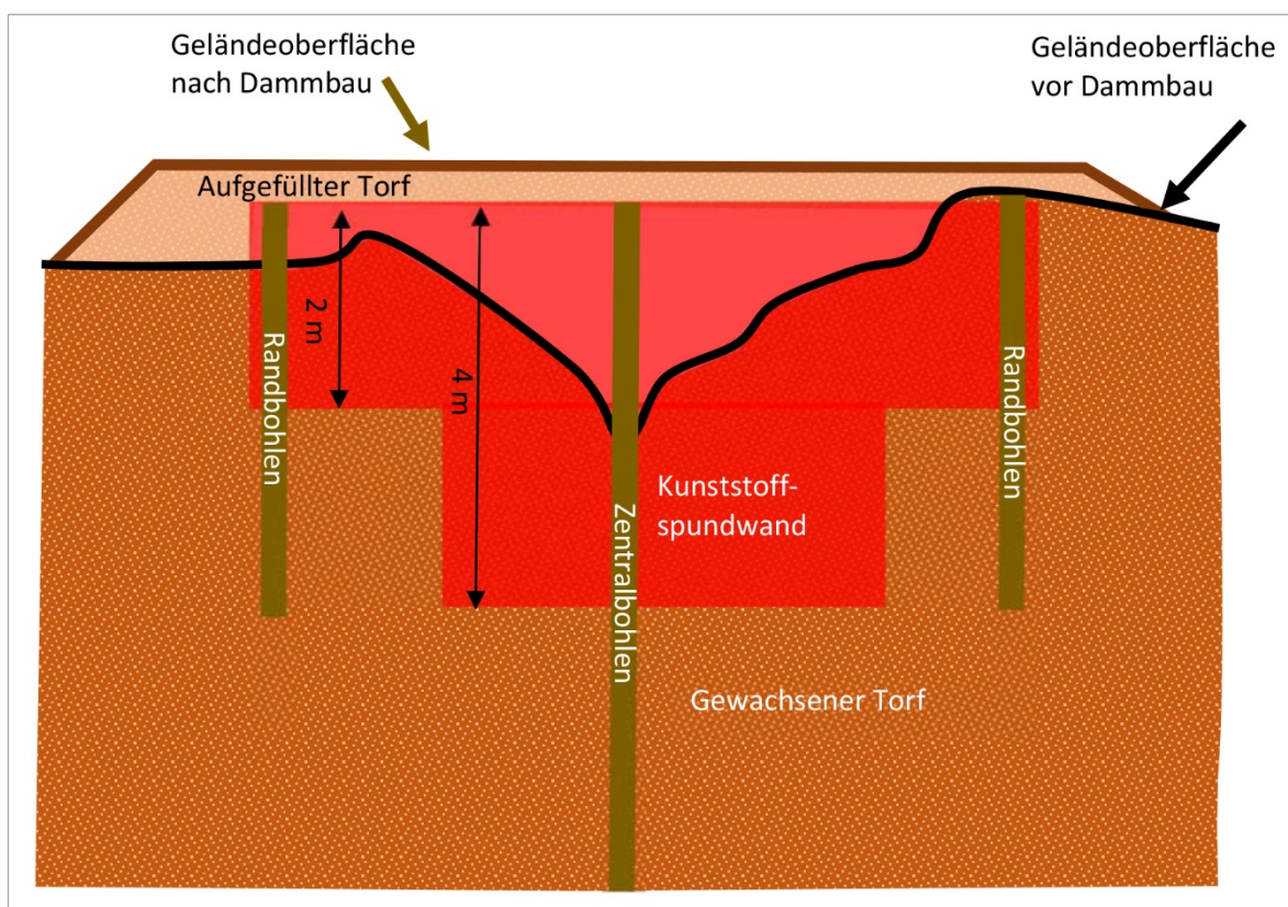
Abb. 4.12: Ausführungsplanung der torfüberdeckten Spundwand, siehe auch Abb. 4.11, rechts (nach KAPFER et al. 2011).
