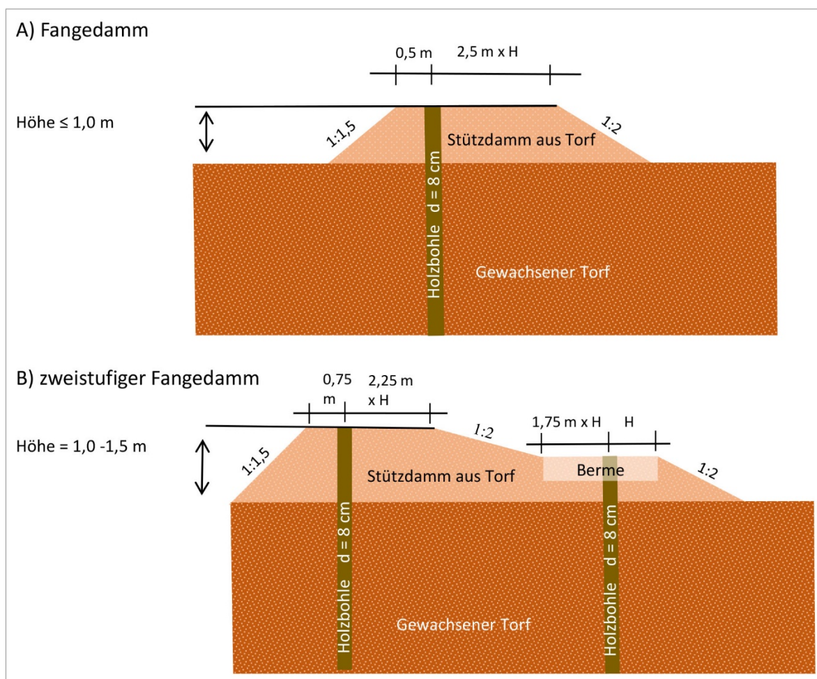
Abb. 4.10: Konstruktion von „Fangedämmen“ im Roten Moor; Wasser steht jeweils links vom Damm (EIGNER & SCHMATZLER 1991).
