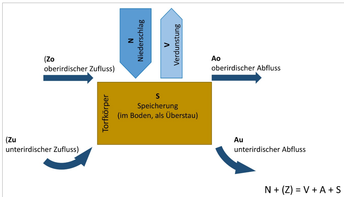
Abb. 2.3: Wasserhaushalt eines Hochmoores.
