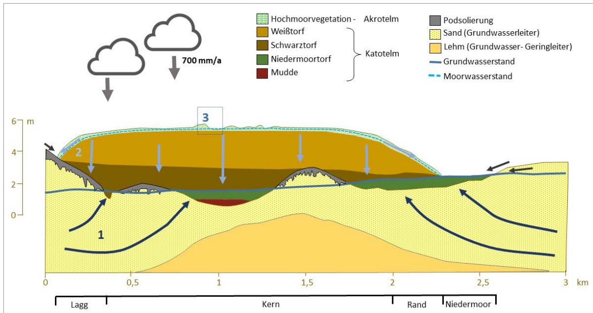
Abb. 2.1 Schema: Landschaftsposition, Wasserhaushalt und Torfbildung prägen die natürlichen Prozesse der Hochmoorbildung (zu den Ziffern 1, 2, 3 siehe nachfolgenden Text). Verändert, nach EGGELSMANN (1990), VAN DIJK et al. (2019), VAN DUINEN et al. (2018).
