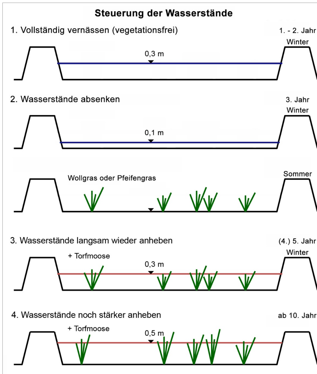
Abb. 5.3: Steuerungsvorschlag der Wasserstände innerhalb der ersten Jahre (verändert, nach MONEY (2004)).
