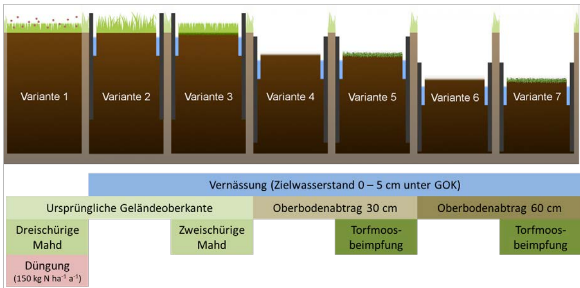
Abb. 6.9: Die Maßnahmenkombinationen der Referenzfläche (Variante 1) und der sechs Wiederherstellungs-Varianten.
