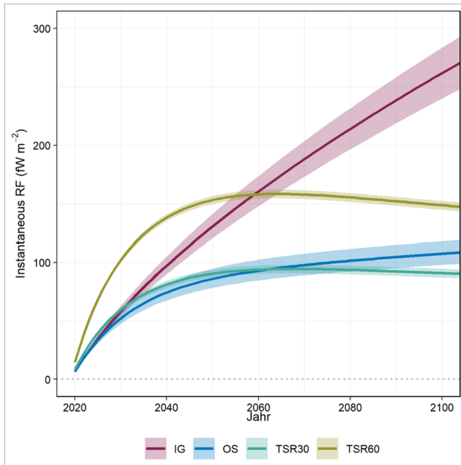
Abb. 6.8: Strahlungsantrieb der OptiMoor-Varianten, wenn man Emissionsfaktoren (IPCC 2014) für die verschiedenen Varianten und die Menge des abgetragenen Oberbodens aus dem OptiMoor-Projekt zugrunde legt (s. HUTH et al. 2021, Table 2), hier dargestellt unter der Annahme einer jährlichen Abbaurate des abgetragenen Oberbodens von 5 % (für höhere und niedrigere Abbauraten s. HUTH et al. 2021). Die entwässerungsbasierte Grünlandnutzung (IG), verglichen mit drei Renaturierungsansätzen ohne Oberbodenabtrag (OS) oder mit ca. 30 bzw. 60 cm Abtrag (TSR30 bzw. TSR60). Die Ansätze mit zusätzlichen Maßnahmen (Torfmoosbeimpfung bzw. Mahd) fehlen, da diese die gleichen Emissionsfaktoren haben, wie die vergleichbaren Varianten. Zuerst publiziert in Restoration Ecology am 22. Juli 2021 (DOI: 10.1111/rec.13490), angepasst von Anke Günther am 13. Oktober 2021.
