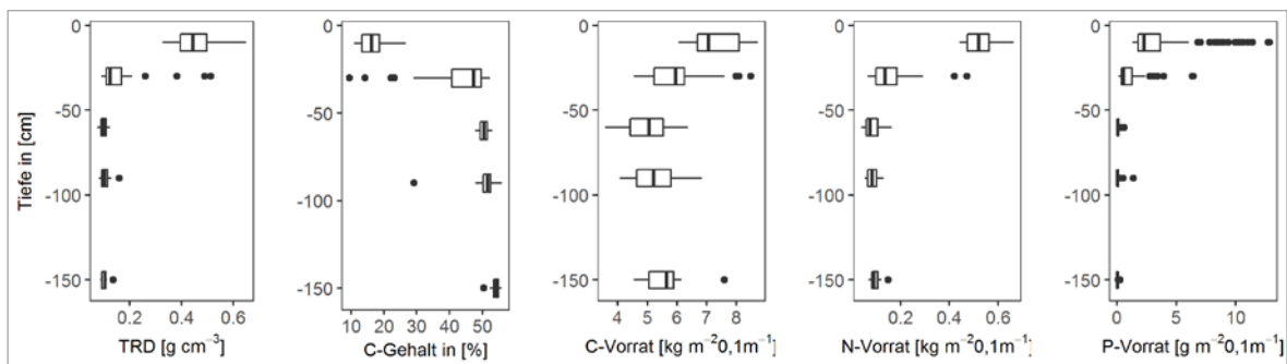
Abb. 6.5: Trockenrohdichte (TRD, in \text{g cm}^{-3} ), C-Gehalt (% der Trockenmasse) sowie Boden-C-, -N- ( \text{kg m}^{-2} 0,1 \text{ m}^{-1} ) und P-Vorräte ( \text{g m}^{-2} 0,1 \text{ m}^{-1} ) im Torfprofil der Versuchsfläche des OptiMoor-Projektes (aus HUTH et al. 2019).
