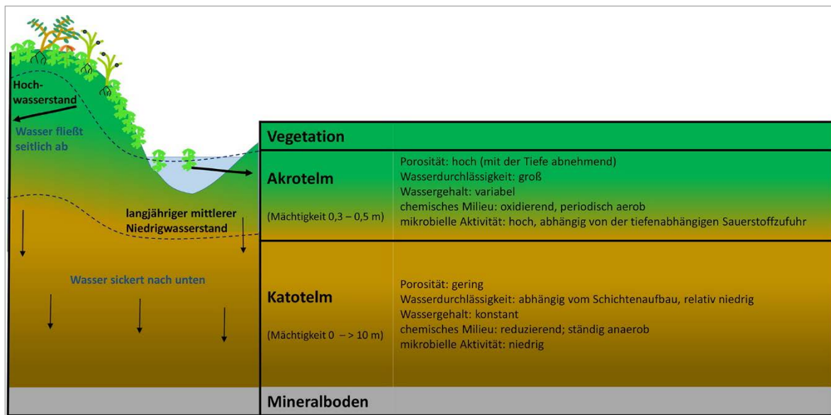
Abb. 2.4: Zweischichtiger Moorkörperaufbau: Akrotelm und Katotelm; geändert, nach SUCCOW & JOOSTEN (2001).
