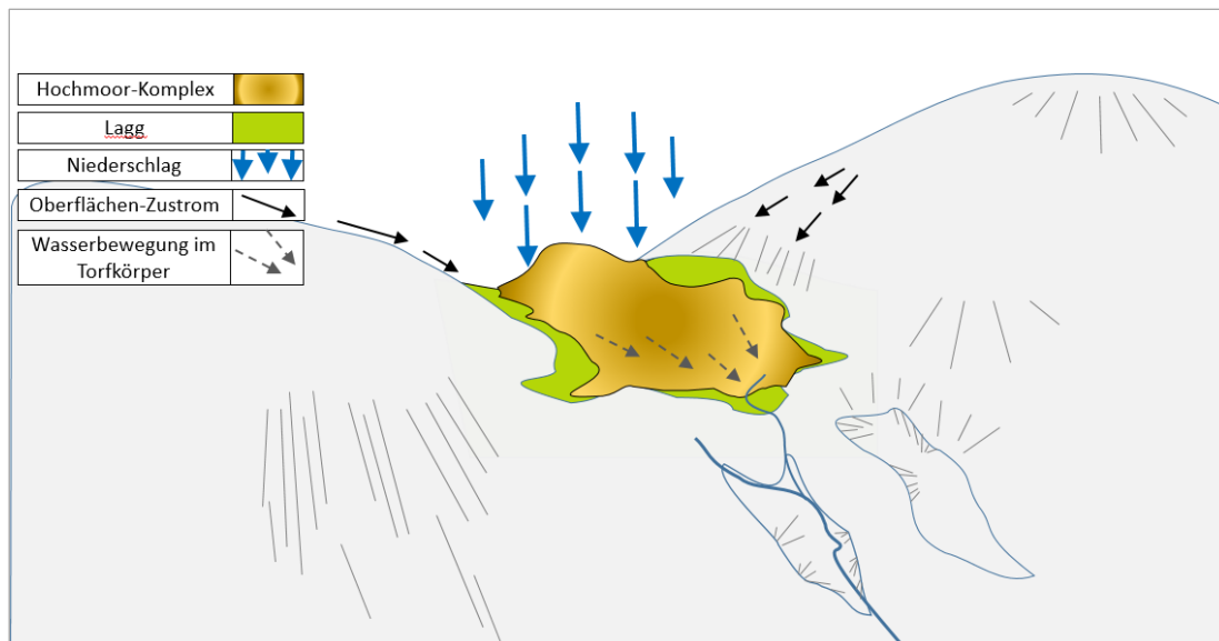
Abb. 7.4: Schematische Darstellung eines Sattelmoores auf einer Wasserscheide (überarbeitet, nach RINGLER & DINGLER 2005). Orange = Torfmoosmoor, grün = mit Grundwasser gespeistes Moor; die Pfeile geben die Herkunft der Speisung (blau) sowie die Strömung von Wasser (schwarz) wieder.
