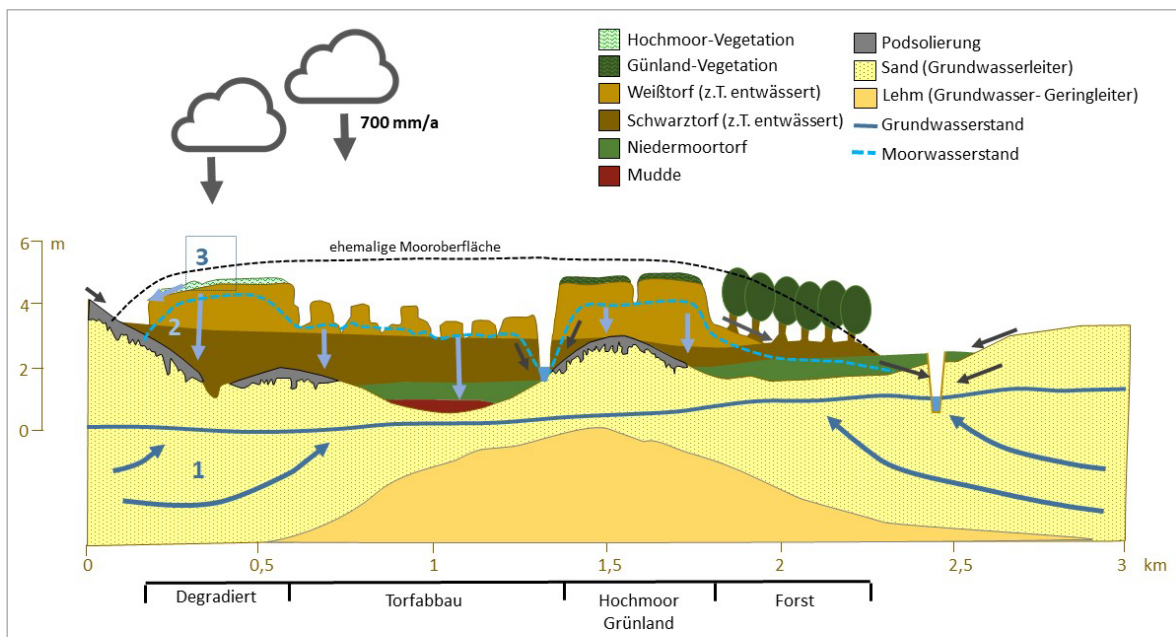
Abb. 2.2: Schema einer degenerierten Hochmoorlandschaft in Folge von Entwässerung und Hochmoor-Nutzung. Wesentliche Veränderungen in Hochmoor- und Landschafts-Wasserhaushalt entstehen durch Fragmentierung des hydraulischen Systems in kleine Einheiten. Die Ziffern 1, 2, und 3 der Abbildung verweisen auf wesentliche Wasserhaushalts-Ebenen von Hochmooren (Erläuterung der Ziffern: siehe nachfolgender Text). Verändert, nach EGGELSMANN (1990), VAN DIJK et al. (2019), VAN DUINEN et al. (2018).
