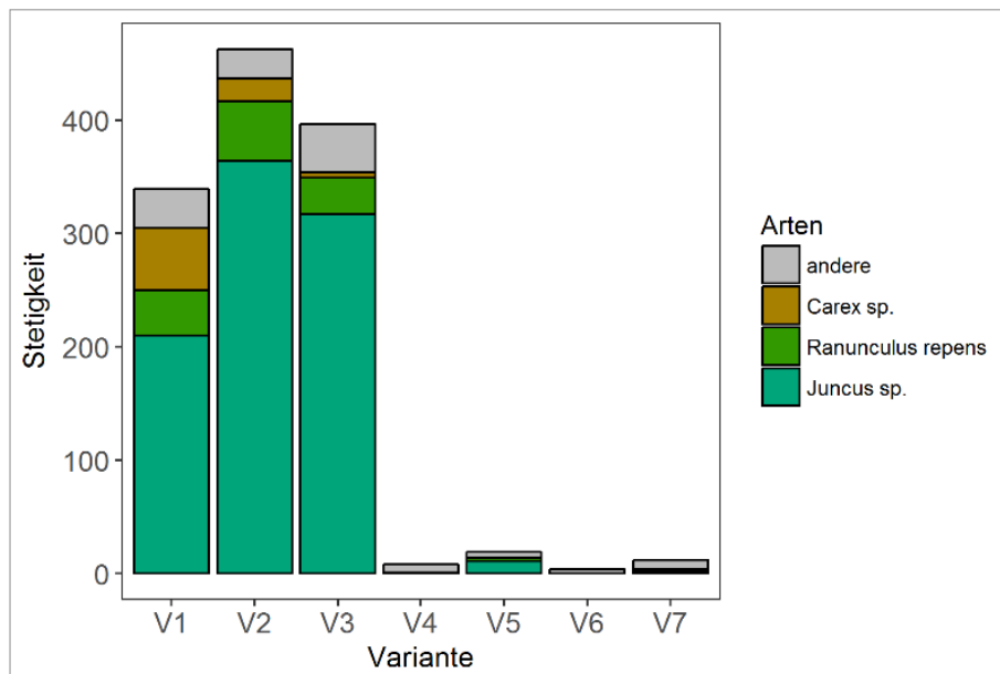
Abb. 6.4: Absolute Stetigkeit der gekeimten Individuen im Torfprofil der Varianten ohne und mit Oberbodenabtrag des OptiMoor-Projektes (HUTH et al. 2019). Die Varianten werden in Abbildung 6.9 beschrieben. Gattungen/Arten mit weniger als 5 % Anteil an der Gesamt-Individuenzahl sind unter „andere“ zusammengefasst.
