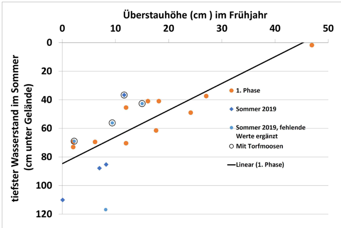
Abb. 5.2: Abhängigkeit der sommerlichen Tiefwasserstände von der winterlichen Überstauhöhe im Leegmoor (negative Zahlen = Wasserstände über Geländeoberfläche; Brux et al., in Vorbereitung).
