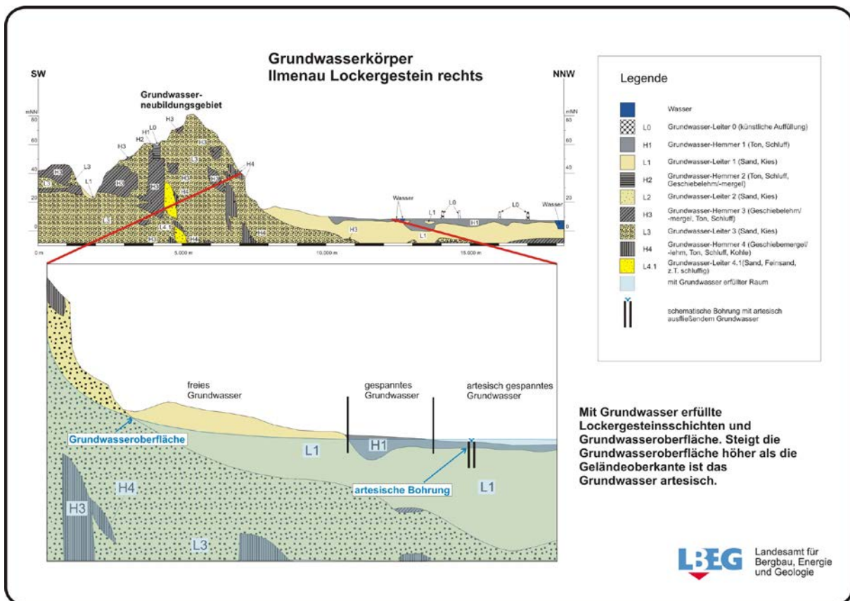
Abbildung 1: schematische Darstellung von artesisch gespannten Bohrlokalationen.
